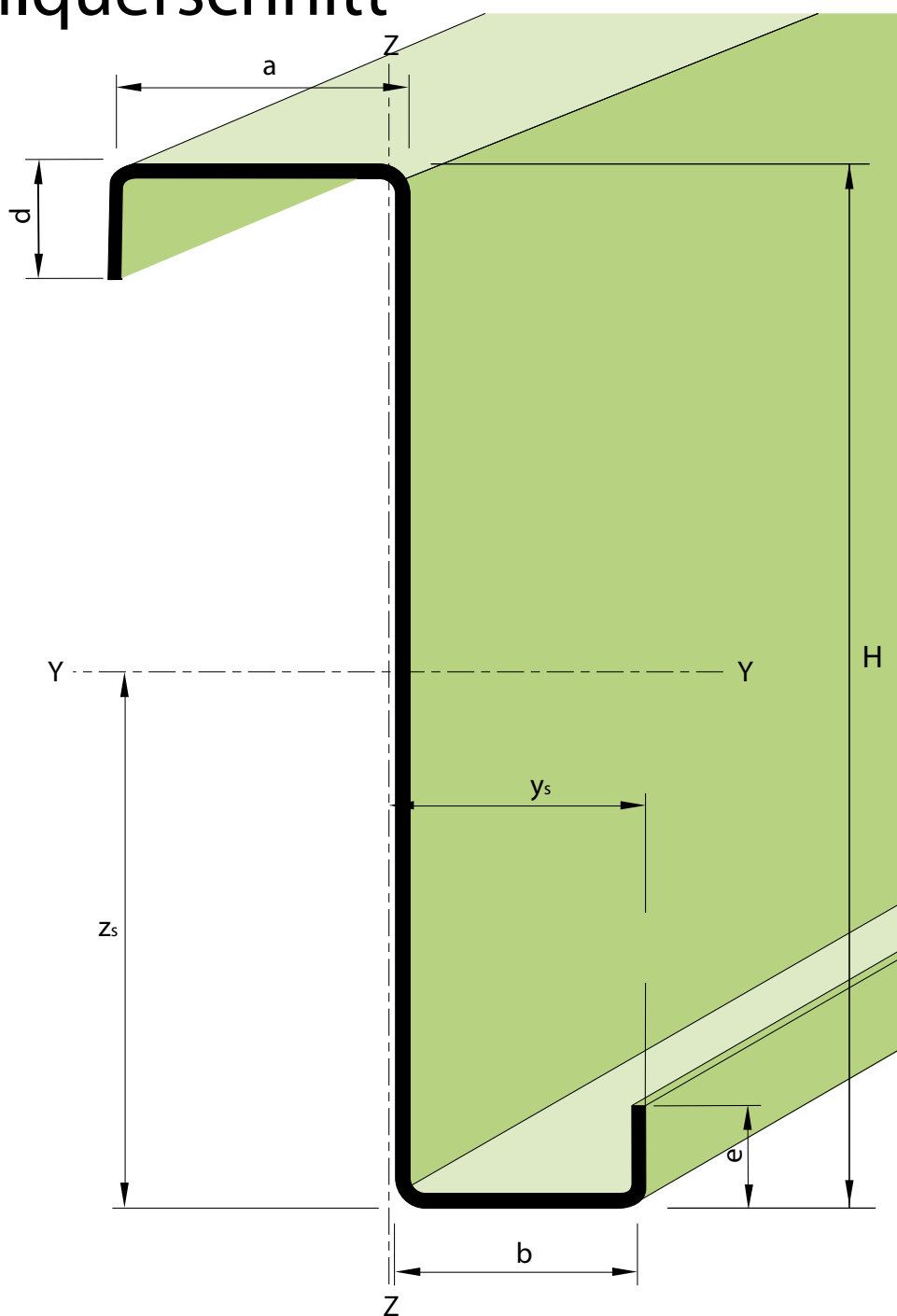
ZED Profilquerschnitt
