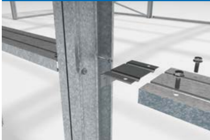
Wandriegel
